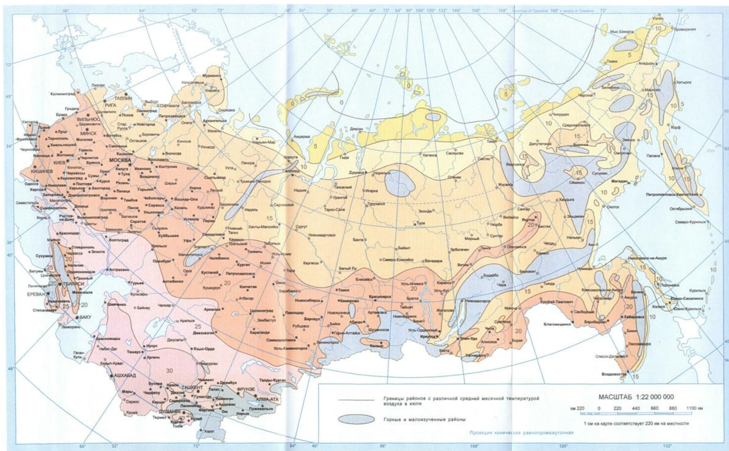
РАЙОНИРОВАНИЕ ТЕРРИТОРИИ СССР ПО ОТКЛОНЕНИЮ СРЕДНЕЙ ТЕМПЕРАТУРЫ ВОЗДУХА НАИБОЛЕЕ ХОЛОДНЫХ СУТОК ОТ СРЕДНЕЙ МЕСЯЧНОЙ ТЕМПЕРАТУРЫ, °С, В ЯНВАРЕ
